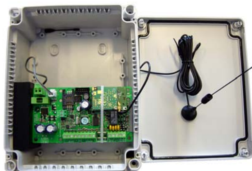
Alpha GSM print + voeding in kast (004497)
